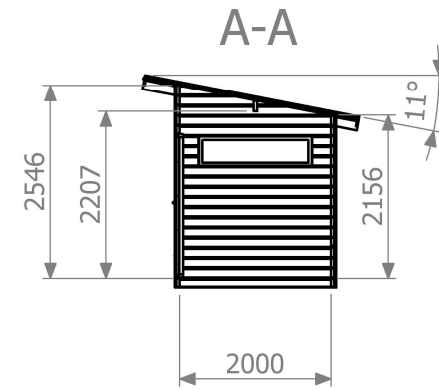
Sektion
