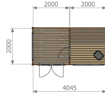
Planritning
