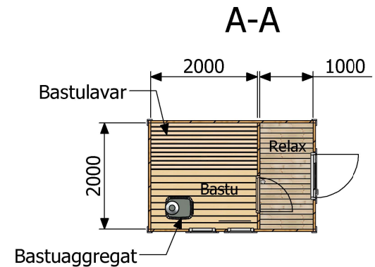
Planritning
