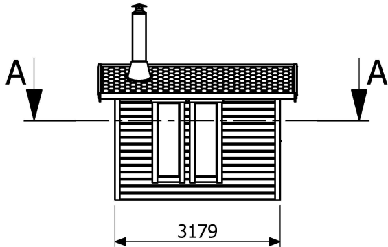
Fasad famsida
