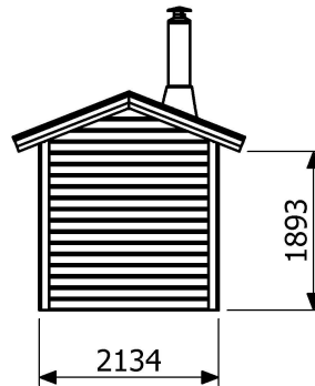
Fasad vänster sida
