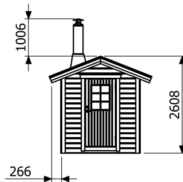
Fasad höger sida
