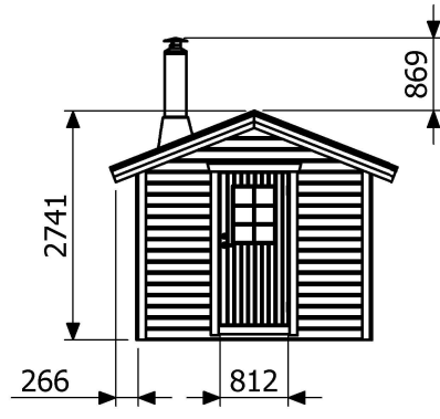
Fasad höger sida
