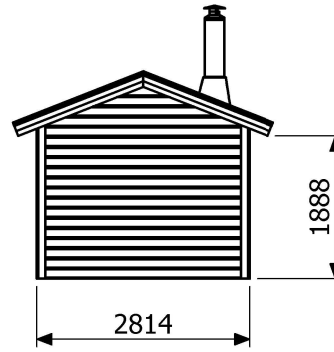
Fasad vänster sida
