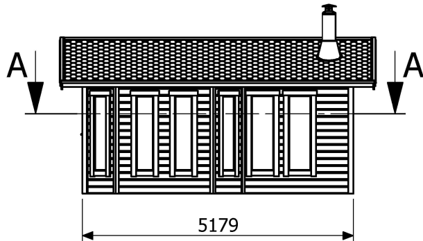
Fasad framsida
