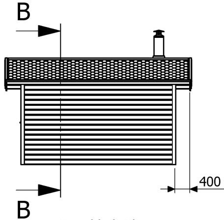
Fasad baksida
