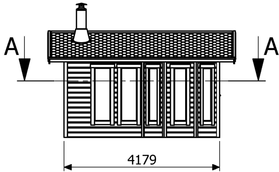
Fasad framsida
