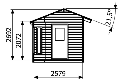
B-B Sektion
