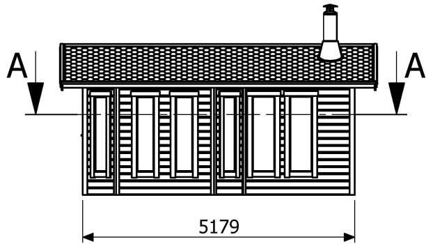
Fasad framsida
