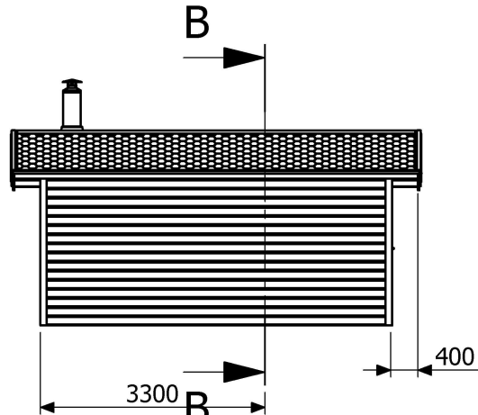
Fasad baksida
