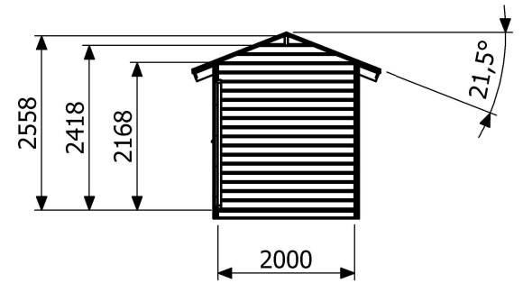
B-B Sektion
