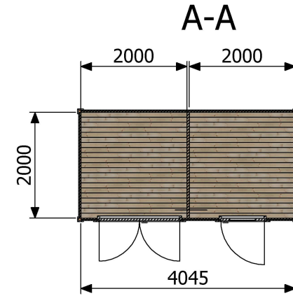
Planritning
