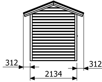
Fasad vänster sida
