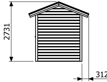
Fasad höger sida
