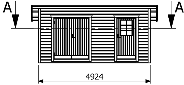
Fasad framsida
