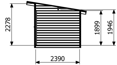
B-B Sektion
