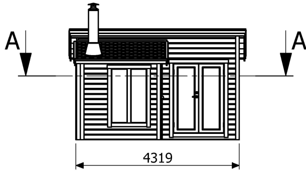
Fasad framsida
