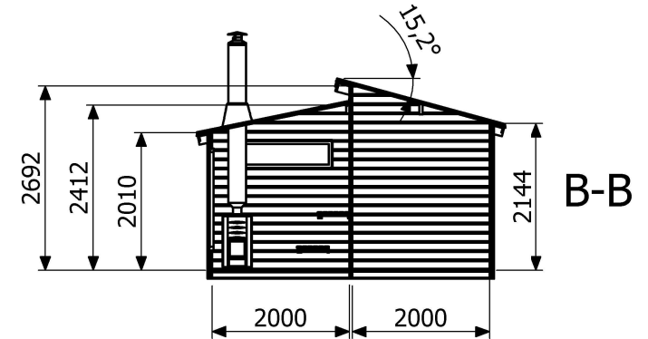
Sektion
