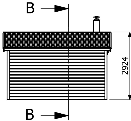
Fasad baksida
