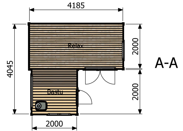
Planritning
