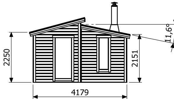
Fasad vänster sida
