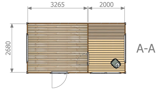
Planritning
