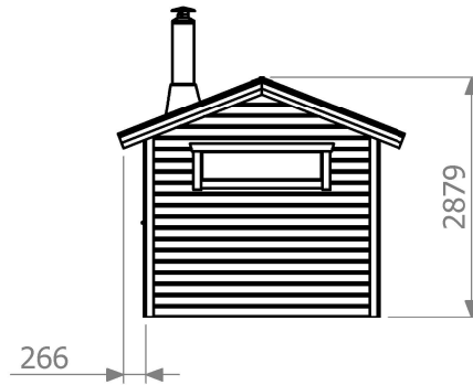
Fasad höger sida
