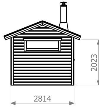
Fasad vänster sida
