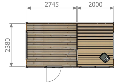
Planritning
