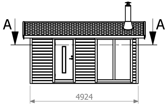
Fasad famsida
