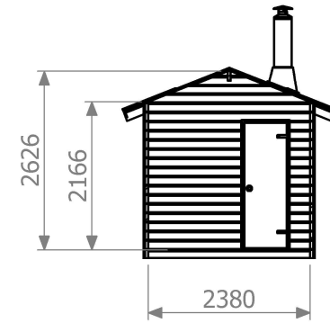
Sektion
