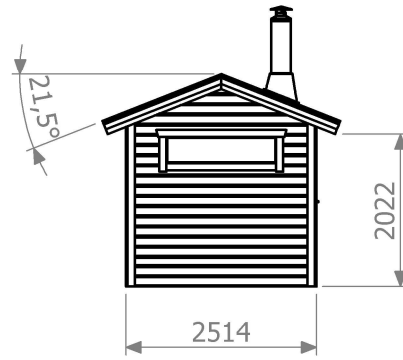
Fasad vänster sida
