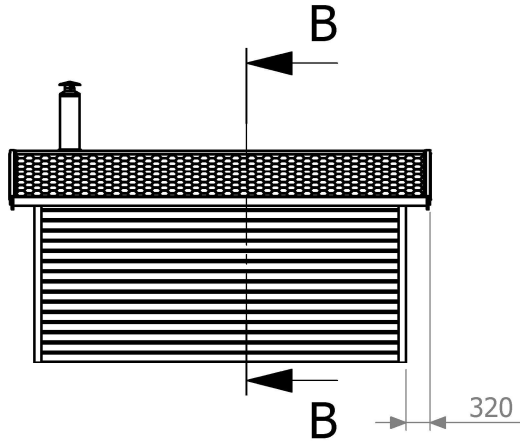
Fasad baksida
