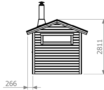
Fasad höger sida
