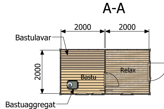
Planritning
