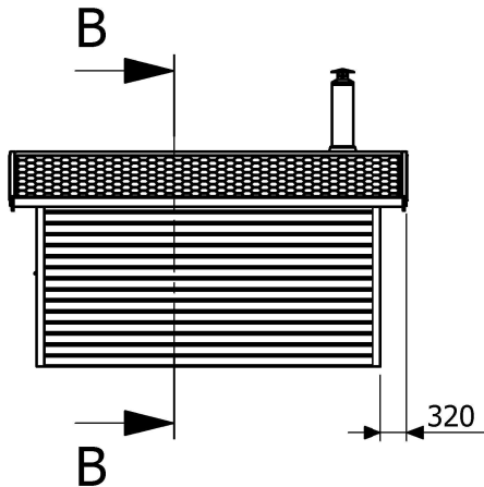
Fasad baksida
