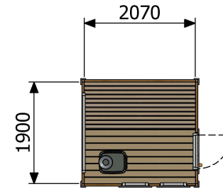
Planritning
