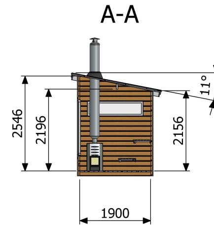
Sektion
