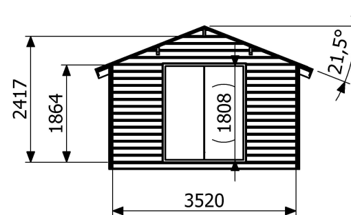
Sektion B-B
