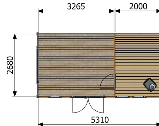
Planritning
