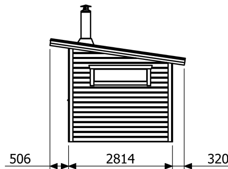
Fasad höger sida
