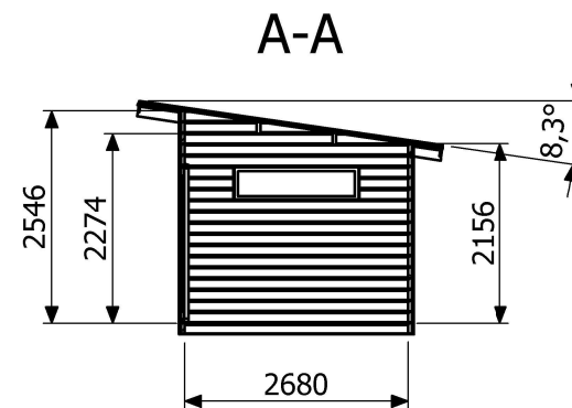
Sektion
